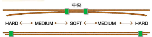
断面図
